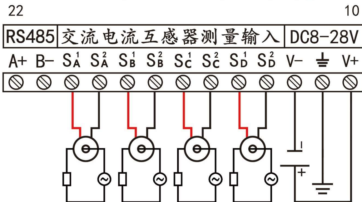
HDXXAXXA5GK-D接线图
