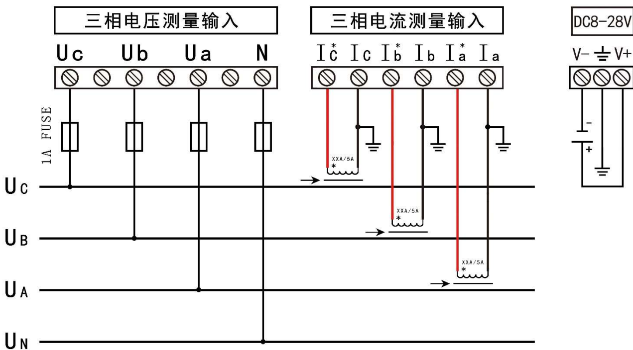
HD250V5A3GK-D接线图
